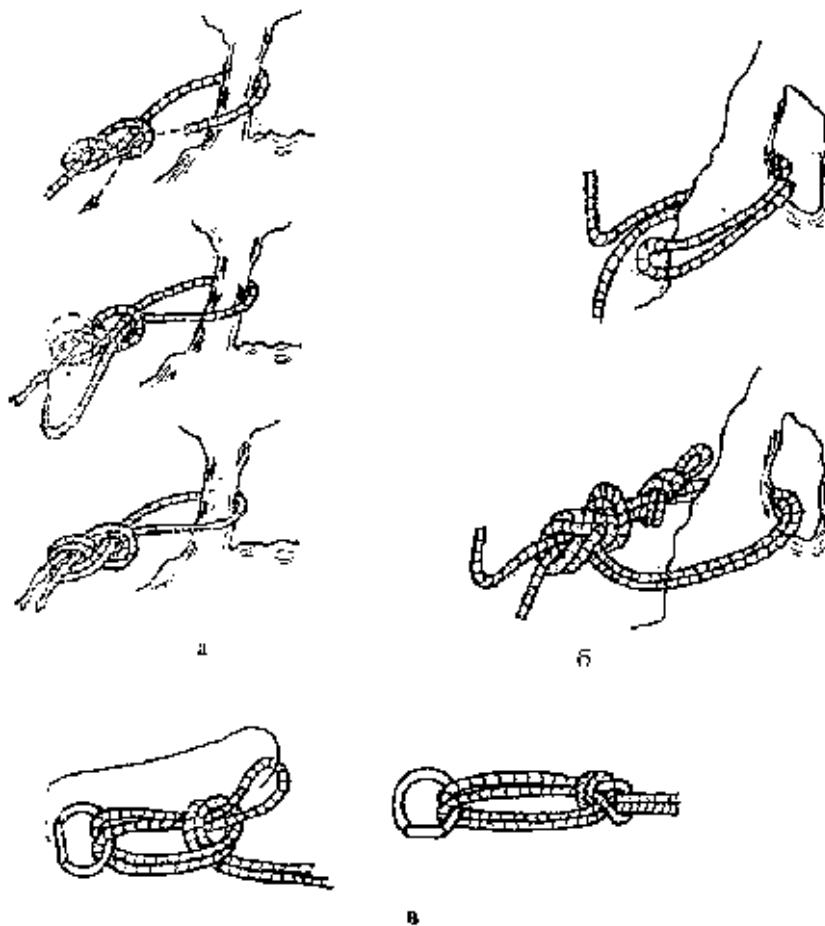
Рис.35. а – восьмерка; б – одинарный булинь на сдвоенной веревке; в – двойной булинь
