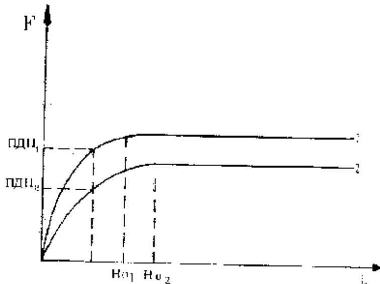
Рис.46. Зависимость ПДН на страховочный ремень от предела Н0: 1 – веревка с меньшим пределом Н0; 2 – веревка с большим пределом Н0
