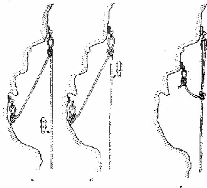
Рис. 14. Устройство основного крепления, расположенного над дополнительным: а, б – неправильно; в – правильно.
