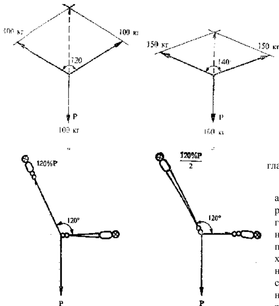
Рис.23. Уменьшение нагрузки на веревку путем ее сдваивания над местом оттяжки
