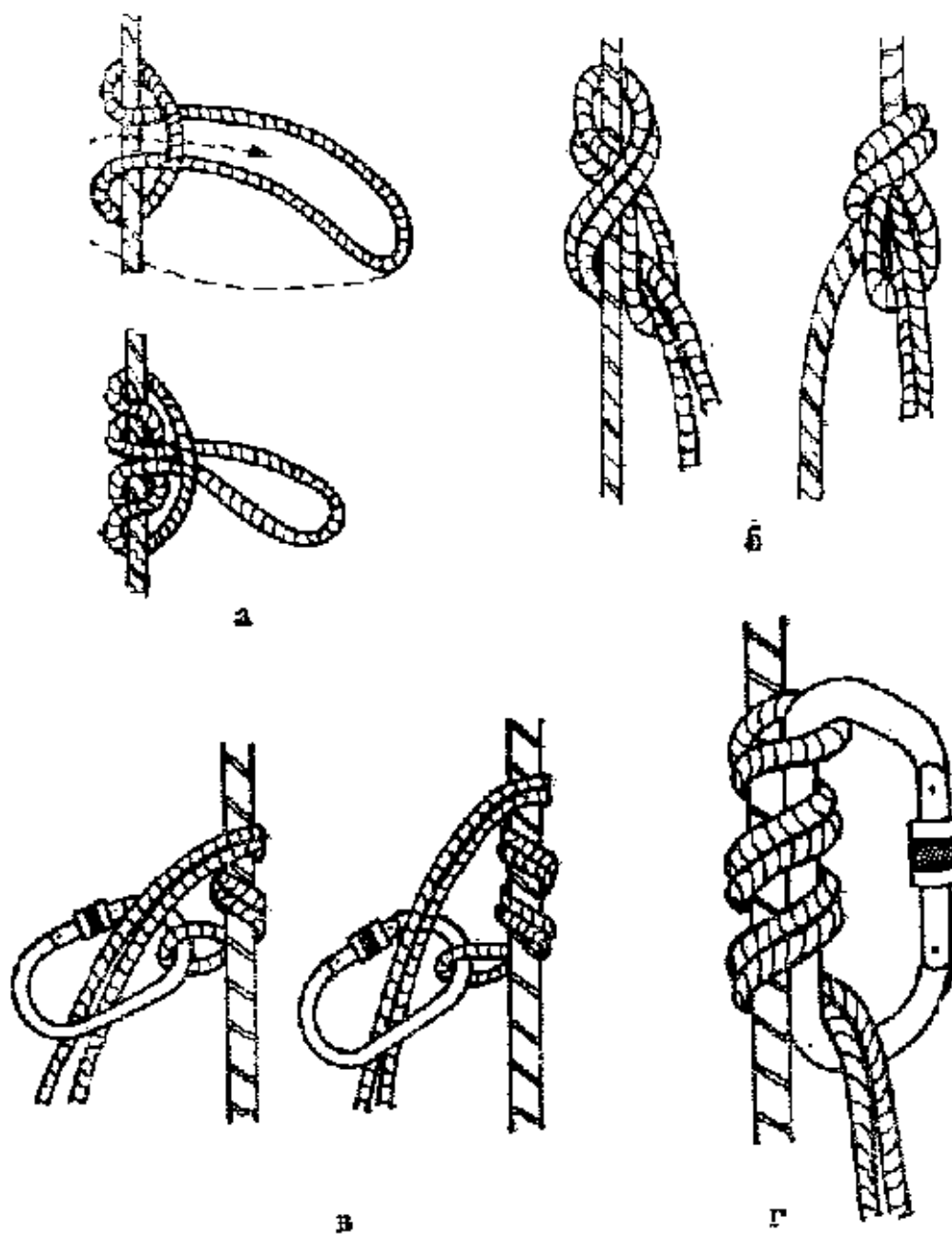
Рис.37. Самозатягивающиеся узлы: а – прусик; б – перекрестный; в – арб; г – бахман
