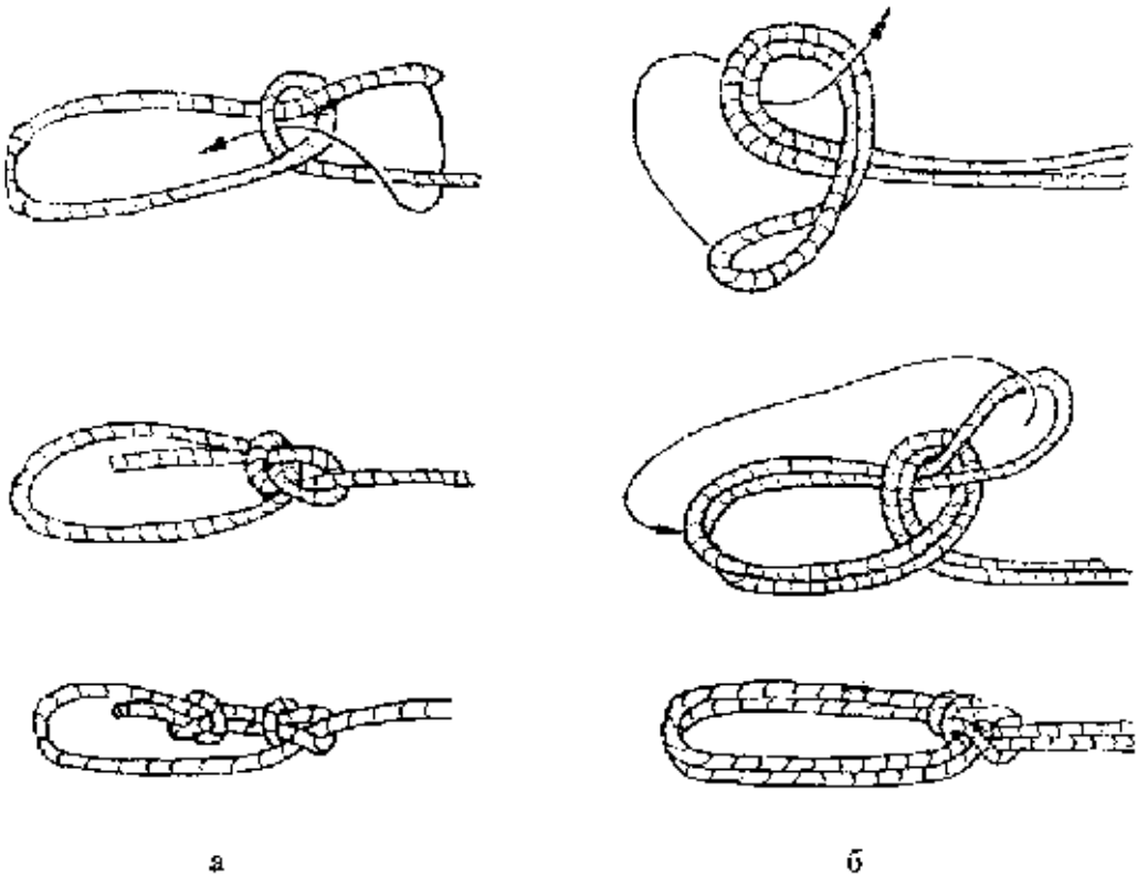
Рис.33. а – одинарный булинь; б – двойной булинь
