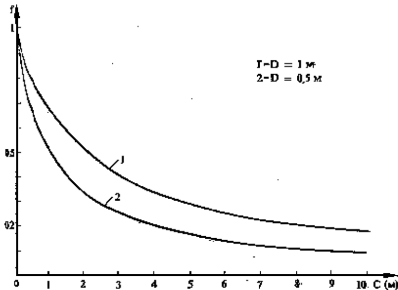
Рис. 29. Зависимость фактора падения от длины веревки над промежуточным креплением C и величины провиса D
