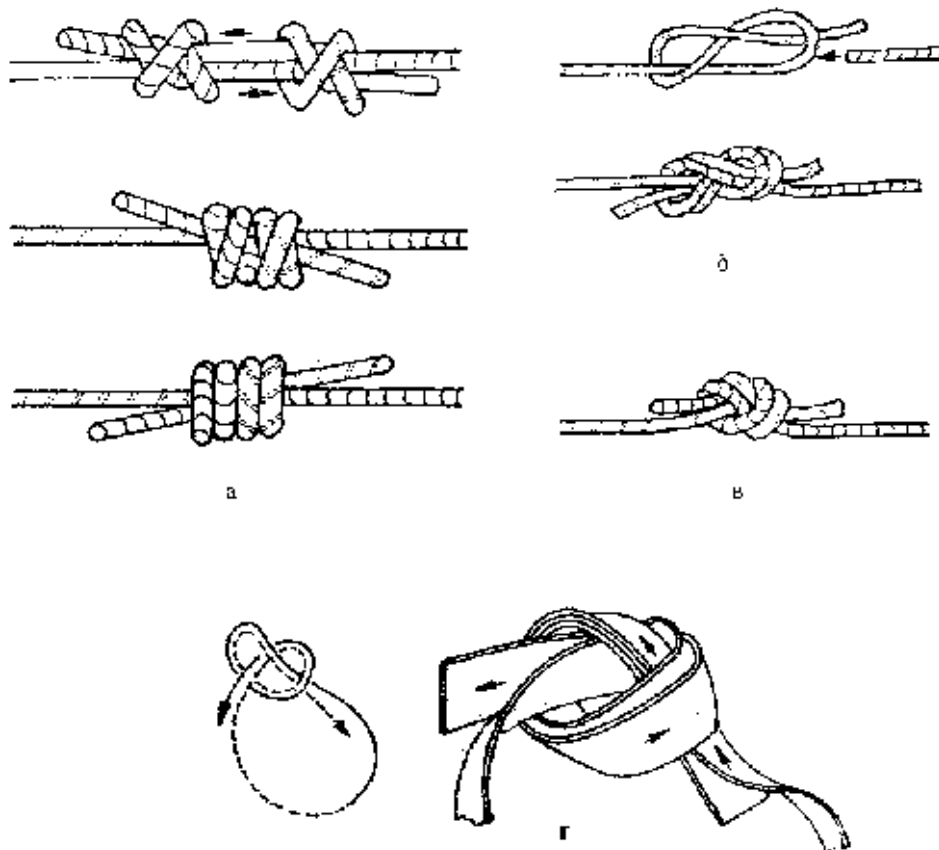
Рис.36. а – двойной ткацкий узел; б – встречная восьмерка; в – встречный проводник; г – ленточный узел
