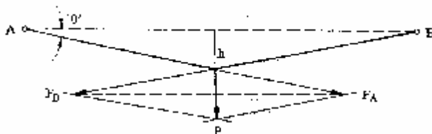
Рис. 21. Силы, действующие на горизонтально натянутую веревку при нагружении.
