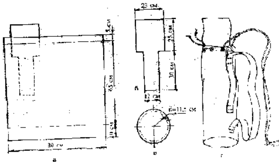
Рис.49. Транспортная сумка: а – выкройка цилиндра (по длинным пунктирным линиям ткань сгибается); б – клапан; в – дно (пришивается к цилиндру по пунктирным линиям); г – общий вид
