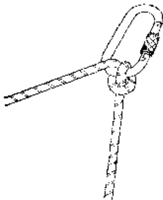
Рис.39. Тормозящий узел
