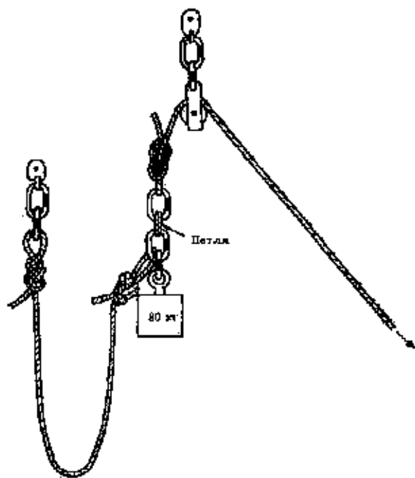
Рис.50. Приспособление для проверки годности статической веревки
