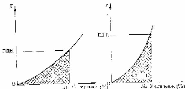
Рис. 2. Удлинение и работа веревки при различной силе нагружения.
