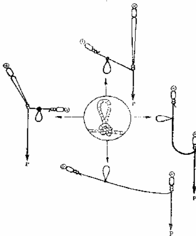
Рис. 16. Амортизирующий узел и схемы креплений, при которых он используется.
