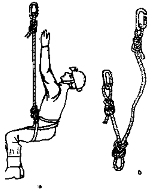
Рис.45. Страховочный ремень: а – неправильно отрегулированный; б – тройкой
