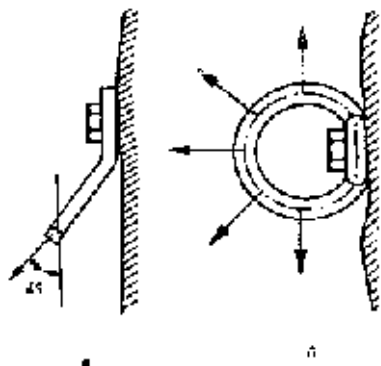
Рис.24. а – профильная планка; б – потолочная планка
