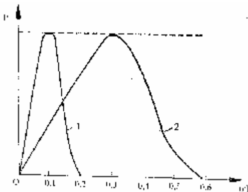
Рис. 5. Длительность импульса силы: 1 — импульс при падении с 1 м с фактором 1; 2 — импульс при падении с 9 м с фактором 1.
