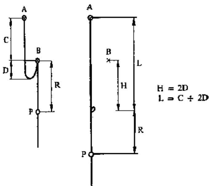
Рис.28. Фактор падения при разрушении
