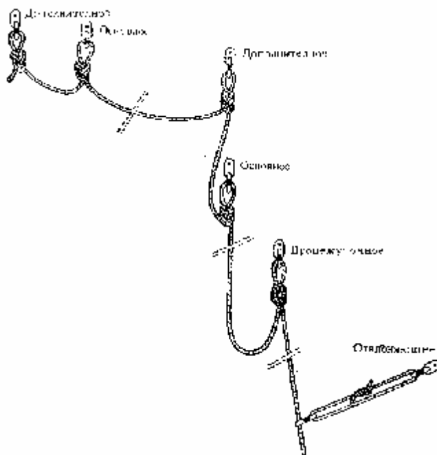
Рис. 10. Виды креплений (дополнительное, основное, промежуточное, отклоняющее).
