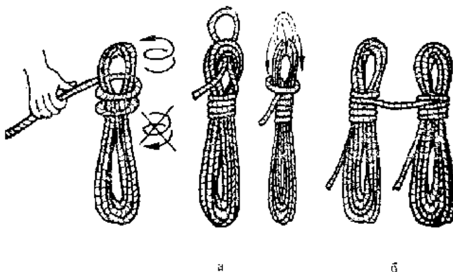
Рис.48. Бухтовка веревки: а – одиночная бухта; б – двойная бухта
