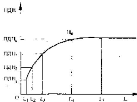
Рис. 12. Зависимость ПДН от длины веревки при одном и том же факторе падения.
